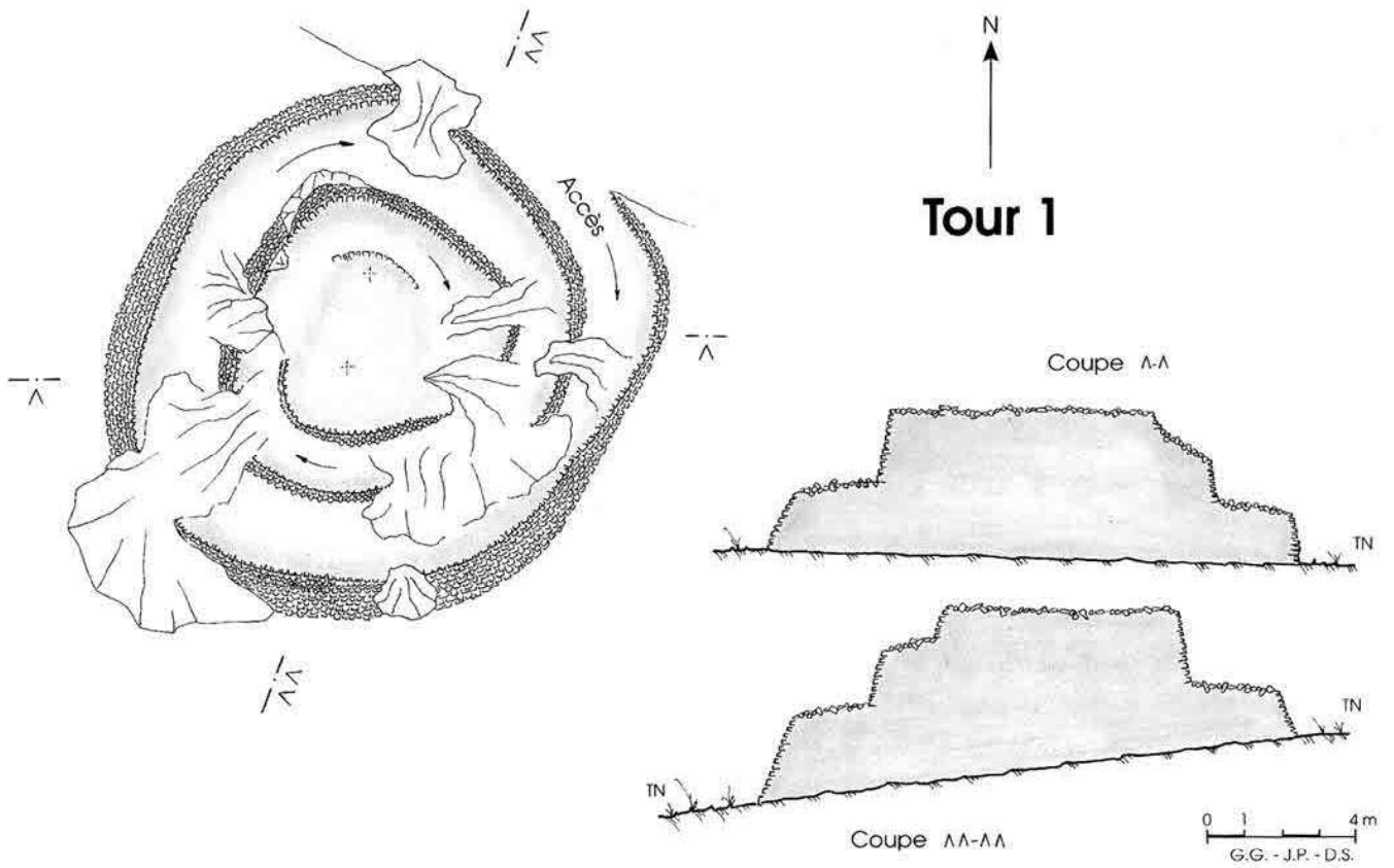
Fig. 3. - Tour 1. Plan et coupes (TN = Terrain Naturel).
