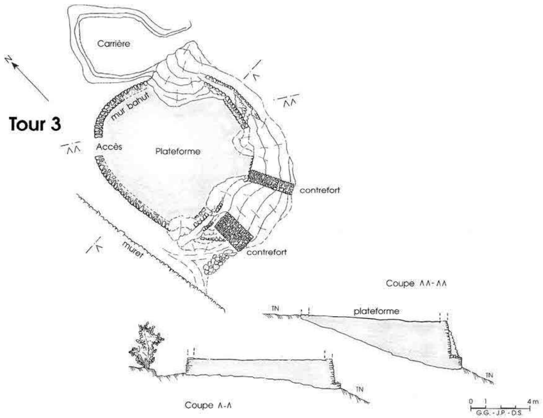
Fig. 7. - Tour 3. Plan et coupes (TN = Terrain Naturel).
