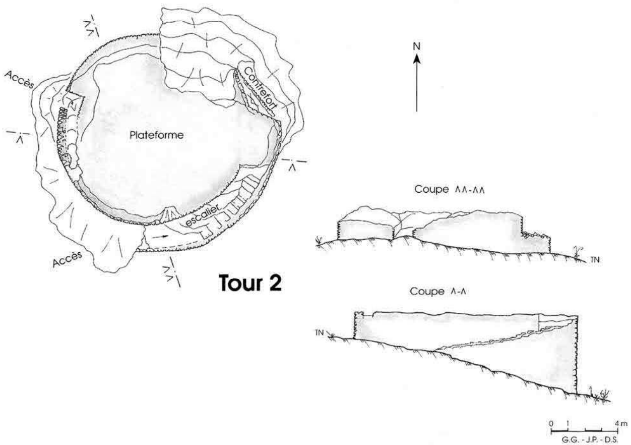
Fig. 4. - Tour 2. Plan et coupes (TN = Terrain Naturel).
