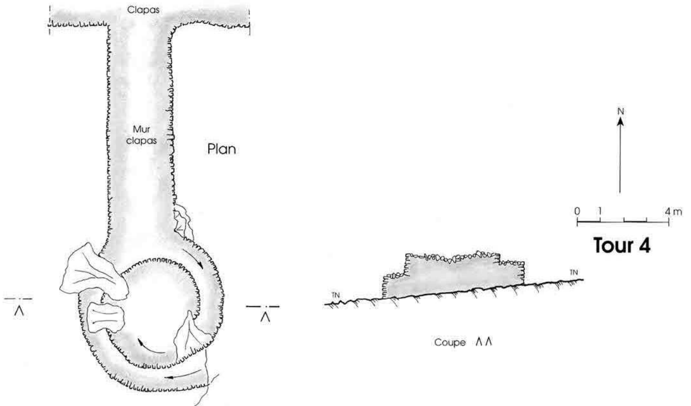
Fig. 8. - Tour 4. Plan et coupe (TN = Terrain Naturel).
