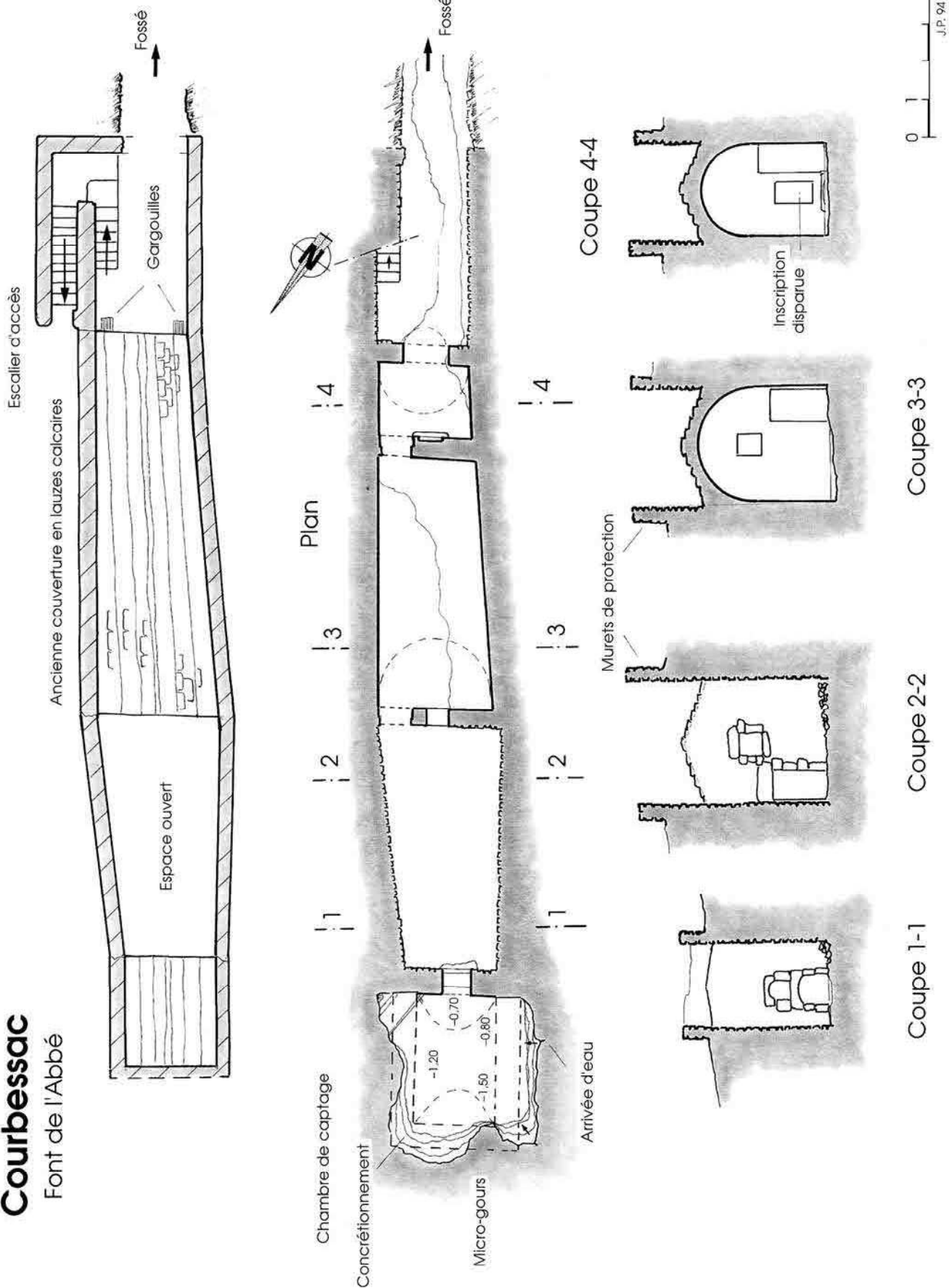
Fig. 15. - Source de la Font de l'Abbé. Plans et coupes (mesures exprimées en mètre).
